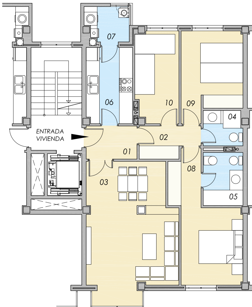
VIVIENDA TIPO DE 3 DORMITORIOS Nº DE VIVIENDAS TOTALES = 16 PORTAL 1 Y 3 . PLANTAS 1ª, 2ª, 3ª, 4ª, 5ª, 6ª, 7ª y 8ª
