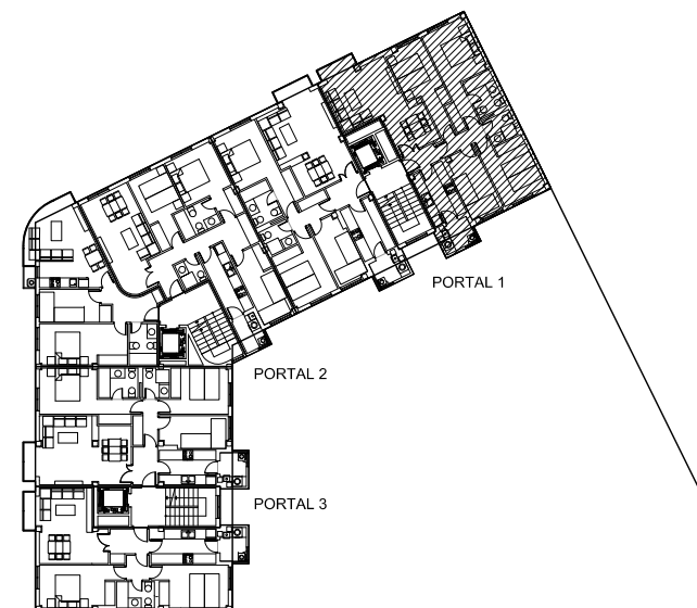
PLANTA TIPO Nº DE PLANTAS TIPO = 8
