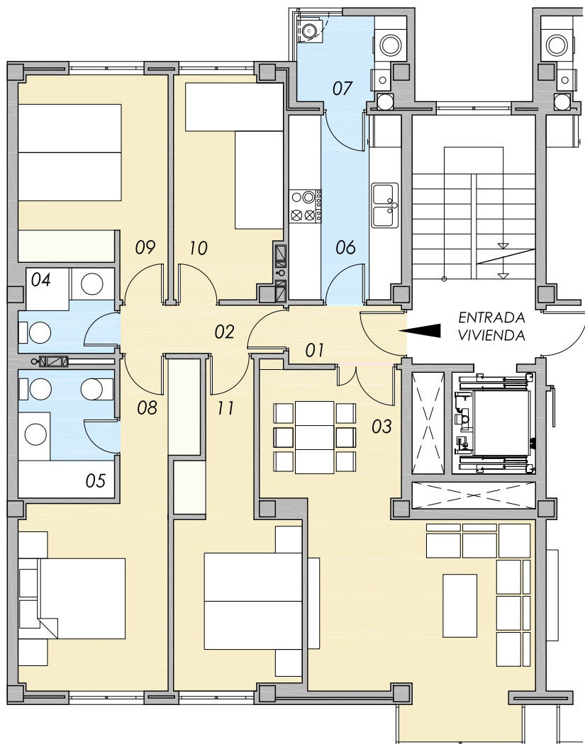
VIVIENDA TIPO DE 4 DORMITORIOS Nº DE VIVIENDAS TOTALES = 8 PORTAL 1 . PLANTAS 1ª, 2ª, 3ª, 4ª, 5ª, 6ª, 7ª y 8ª
