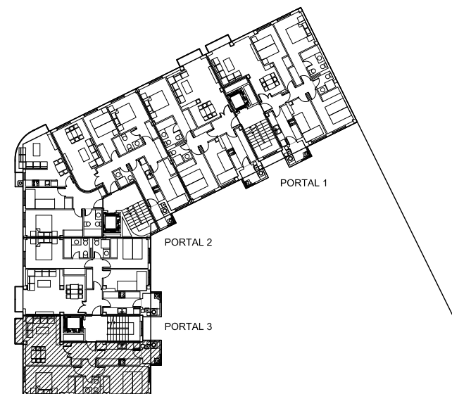
PLANTA TIPO N° DE PLANTAS TIPO = 8
