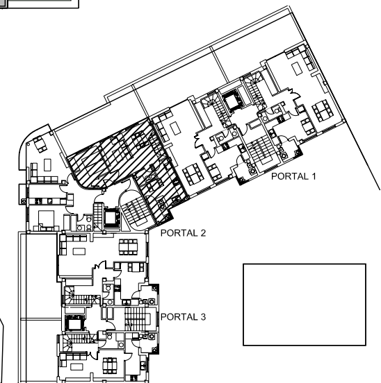
PLANTA 2ª DEL DUPLEX
