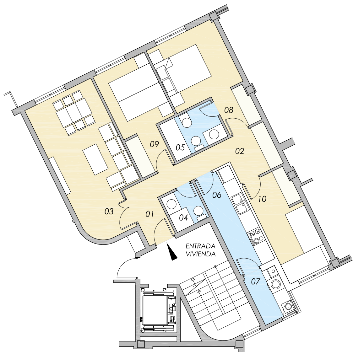
VIVIENDA TIPO DE 3 DORMITORIOS Nº DE VIVIENDAS TOTALES = 8 PORTAL 2 . PLANTAS 1ª, 2ª, 3ª, 4ª, 5ª, 6ª, 7ª y 8ª
