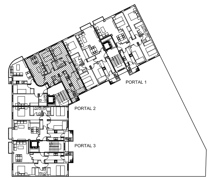
PLANTA TIPO Nº DE PLANTAS TIPO = 8
