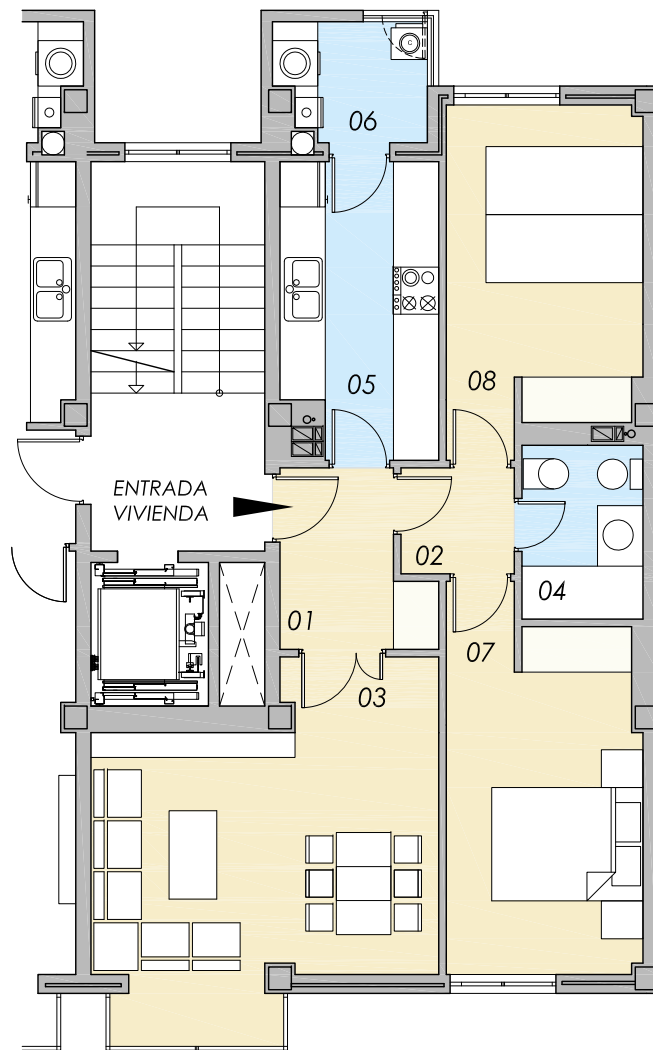
VIVIENDA TIPO DE 2 DORMITORIOS N° DE VIVIENDAS TOTALES = 8 PORTAL 3 . PLANTAS 1ª, 2ª, 3ª, 4ª, 5ª, 6ª, 7ª y 8ª
